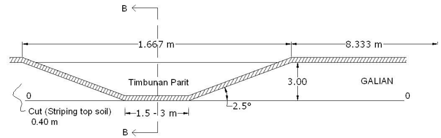
Penampang A-A
