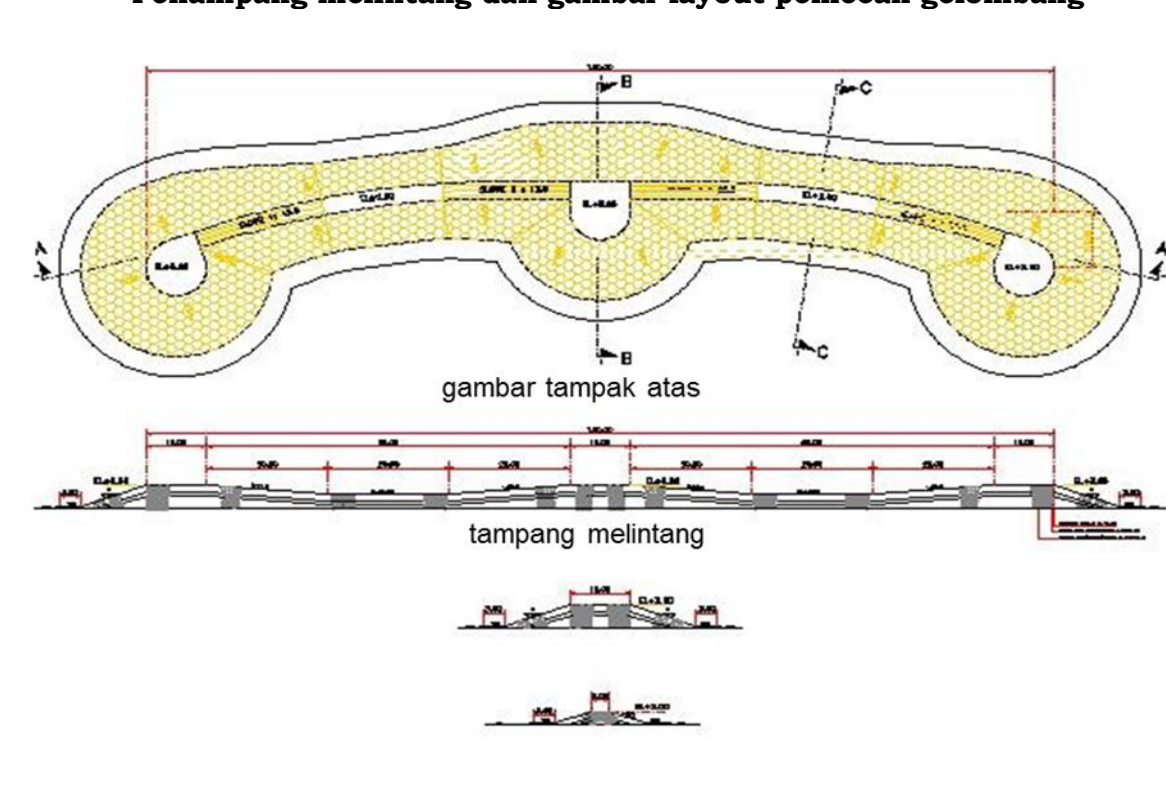
Gambar II.F.23 Denah dan tampang melintang konstruksi pemecah gelombang
