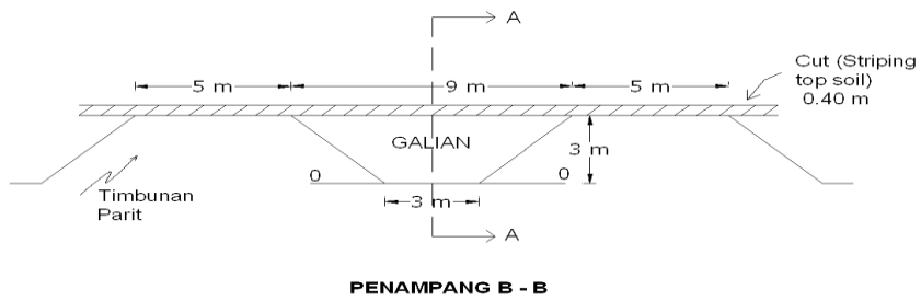
Penampang B-B
